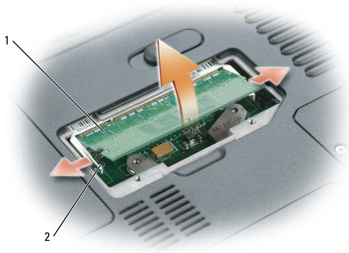
1 内存模块
