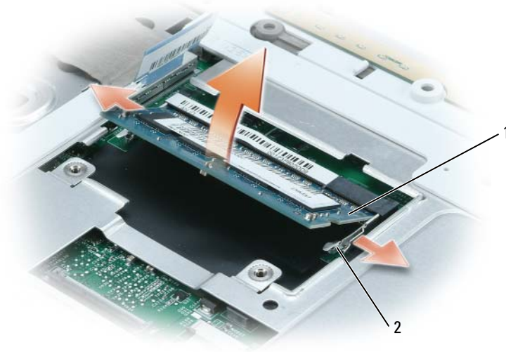
1 内存模块
