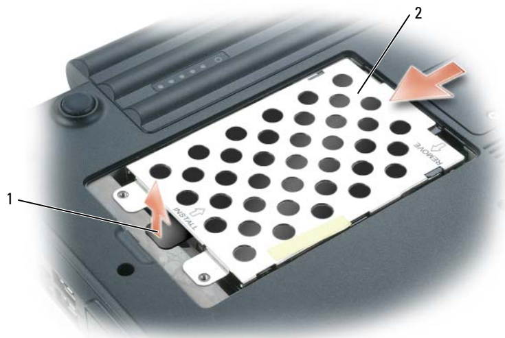
1 推拉卡舌
