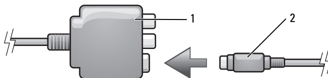
1 复合视频适配器 2 S-video 电缆
