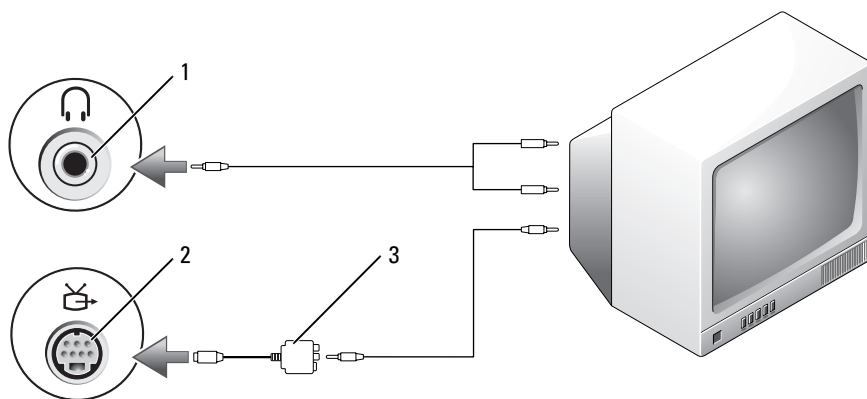
1 音频输入连接器 2 S-video 电视输出连接器 3 复合视频适配器
